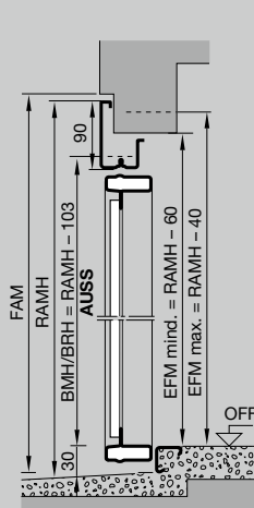
Dübelmontage mit unterem Anschlag
