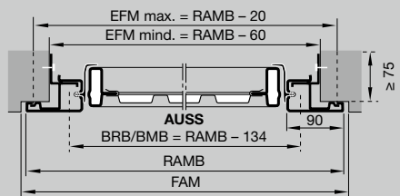
Klemmontage (mind. 50 mm, max. 100 mm Laibungstiefe)
