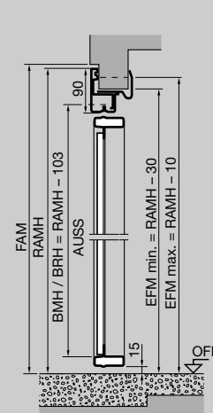
Klemmontage ohne unteren Anschlag
