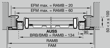
Klemmontage (mind. 50 mm, max. 100 mm Laibungstiefe)
